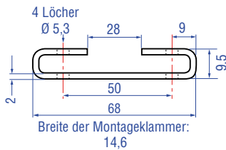
Montageklammer Artikelnr. 403 508
