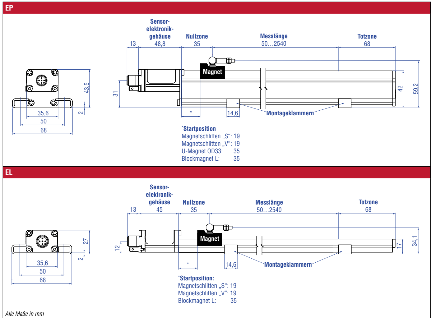
Abb. 3: Temposonics® EP/EL mit Magnetschlitten
