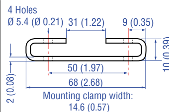
Montageklammer Artikelnr. 403 508
